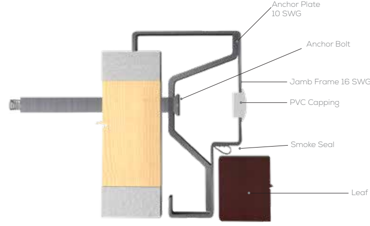
METAL JAMB FRAME
