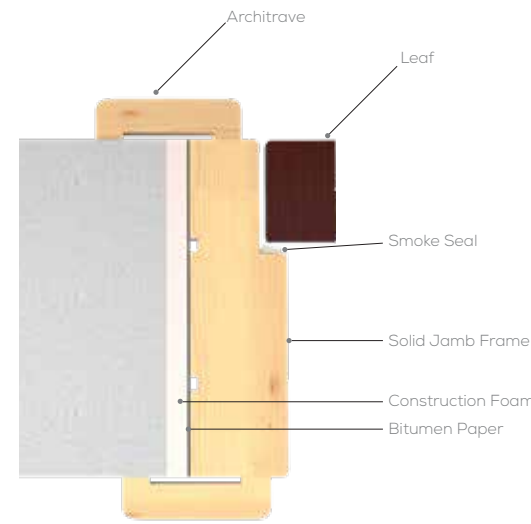
SOLID JAMB FRAME
