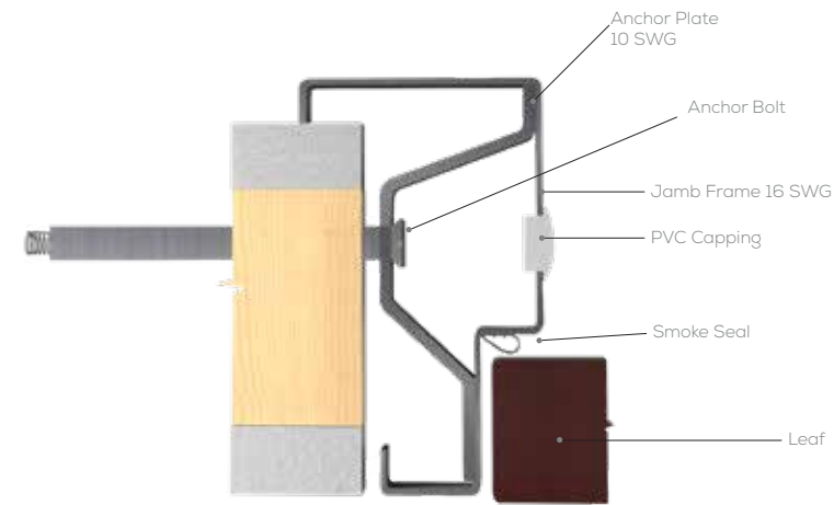
METAL JAMB FRAME
